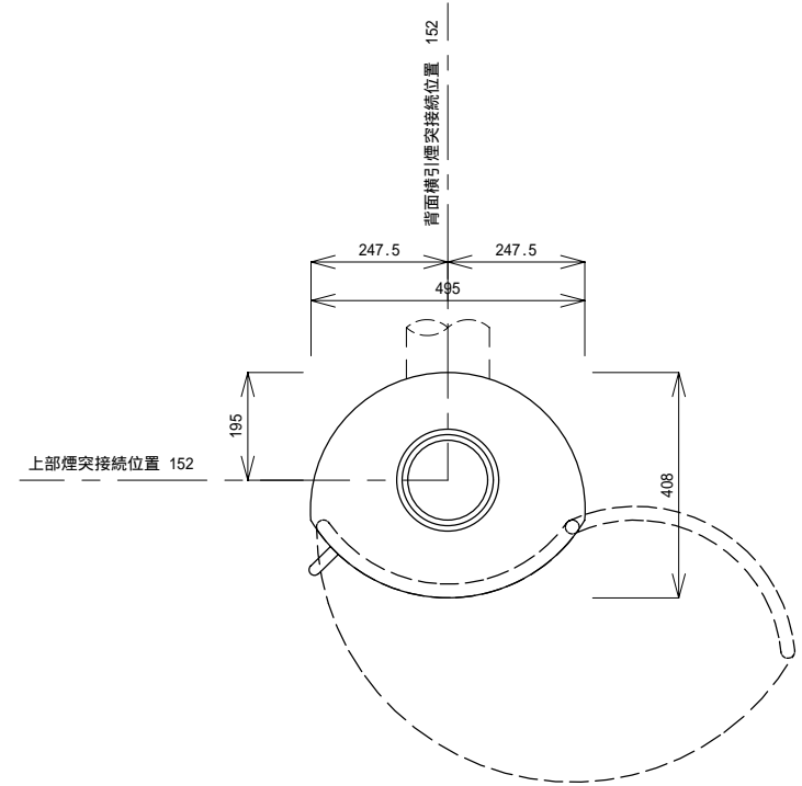
平面図
