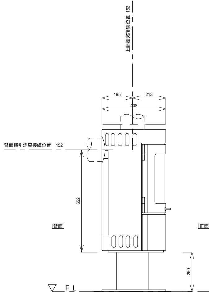
側面図
